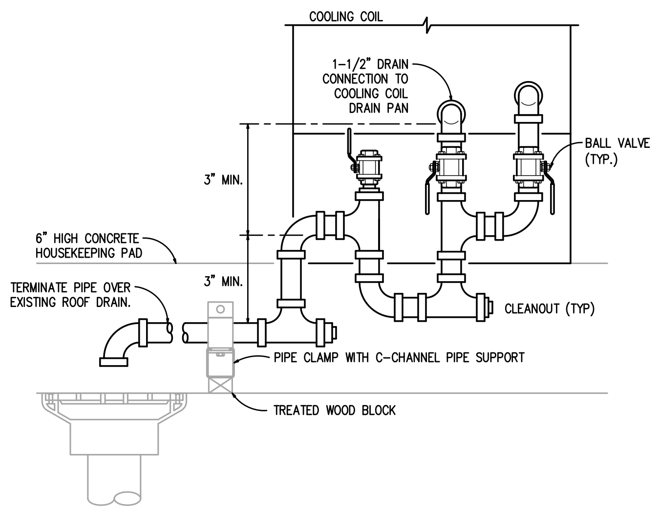
2 DRIP PAN DRAIN DETAIL SCALE: N.T.S.
